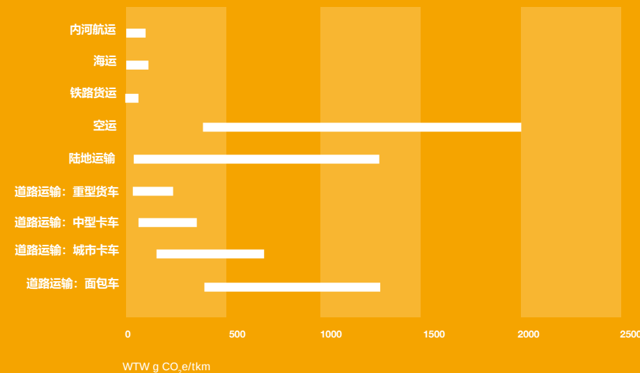
图 1 根据2019年GLEC默认因子，不同类型货物运输WTW排放强度值的示例
