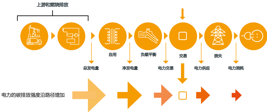
图 1 上游活动到最终消耗的碳强度 (Moro & Lonza, 2018)
