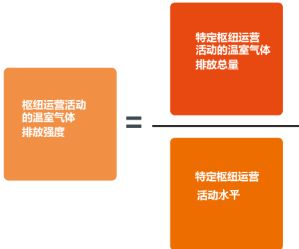
图 3 计算枢纽活动类别的排放强度（HOCs）
