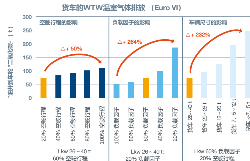
图 4 空驶率、负载率和车辆尺寸对排放的影响 26
