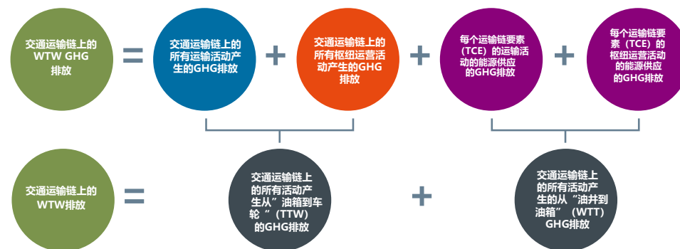
图 4 GHG “油井到车轮”（WTW）排放
